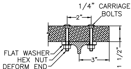
SECTION A-A - LEG & SLAT
